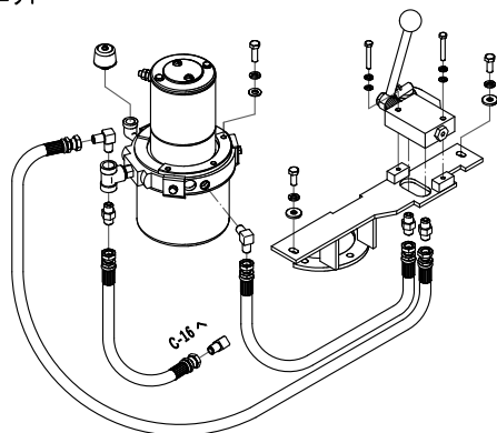
H : 油圧ユニット
