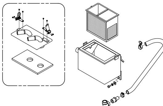
K : バキュームタンク
