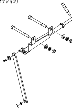
F : コントロール デロック機構 (オプション)
