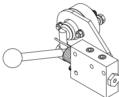
4500-H1-0005 油圧昇降レバーブロック (DBS仕様) 完成図
