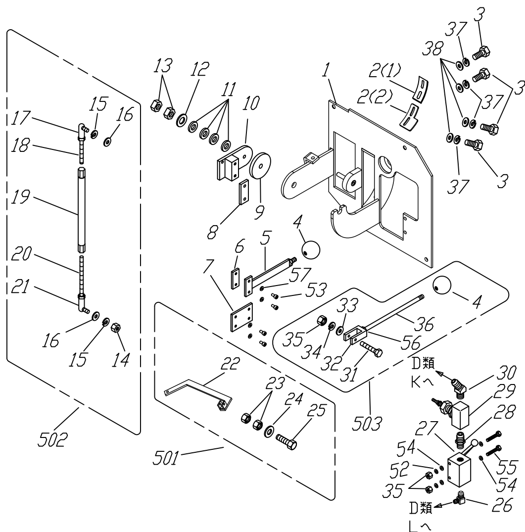
デフロック機構 オプション
